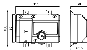
Steuerbox
