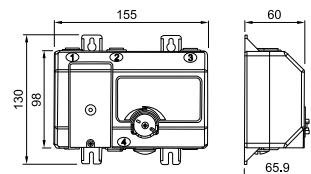
Steuerbox
