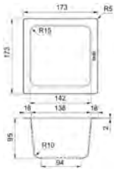
Kleiner Restbehälter
