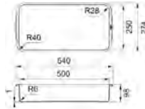
Aufbewahrungsschale
