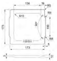
Bambus Verschlussdeckel
